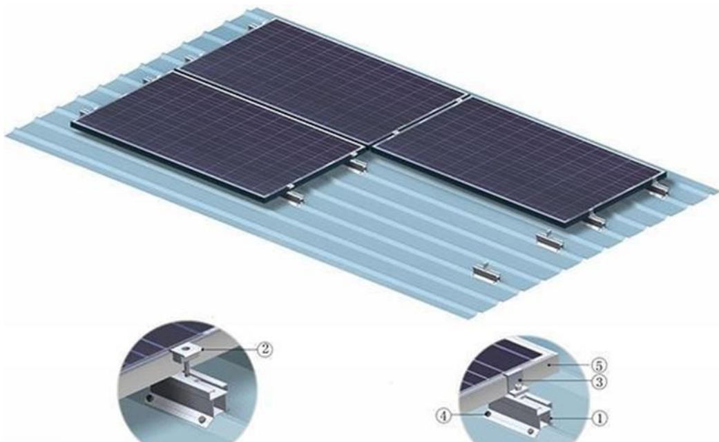
Slika 12: Prikaz montiranja
