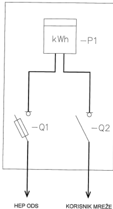
Slika 6. Prikjučno mjerni ormar (PMO) za 1 OMM, smjer proizvodnje: P \leq 50 kW, smjer potrošnje: P \leq 50 kW (izravno mjerenje) – za sunčane elektrane
