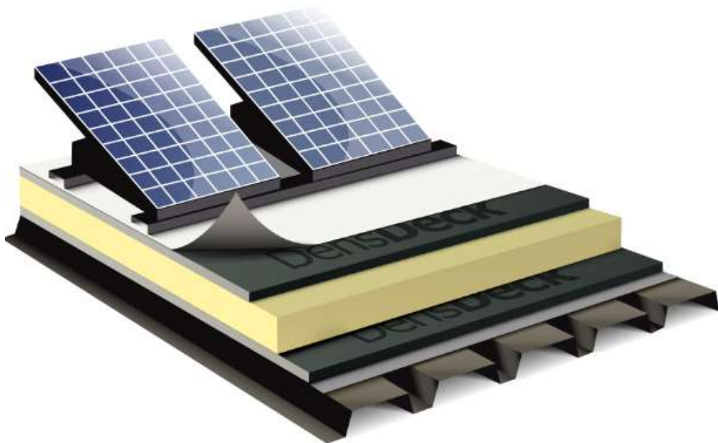
Slika 12: Prikaz montiranja
